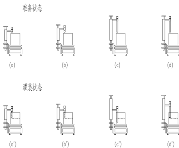
图A.1 4种灌装型式示意图
